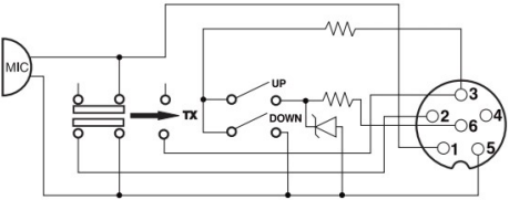
PRISE MICRO À 6 BROCS HES • CONEXIÓN DEL MICRO 6 PINS 6-PIN MICROPHONE PLUG • WTYK MIKROFONU 6-PIN
