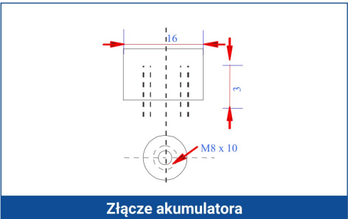
Złącze akumulatora
